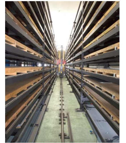
▲自動倉庫内
